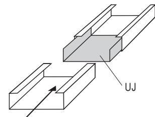
Säleiden jatkaminen UJ-jatkoskappaleilla.
