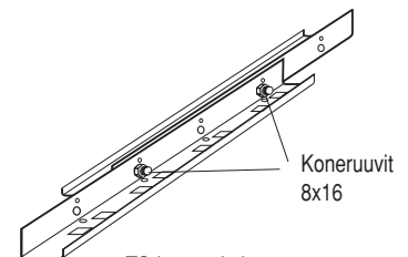
TS-kannattimien jatkaminen liittimillä
