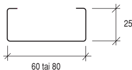
KPR-60 tai KPR-80-säle
