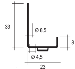
TS-kannatinkiskojen ja ripustusreikien mitoitus
