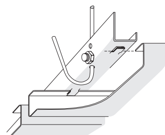
Sälekaton reuna CLL-3048-kaksoiskulmalistalla.
