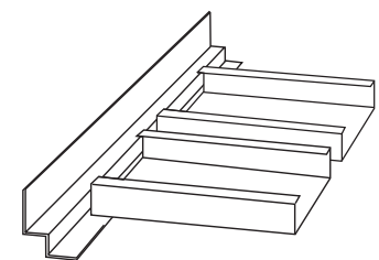
Sälekaton reuna CLL-3048-kaksoiskulmalistalla.
