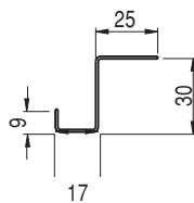
Kannatinlista
