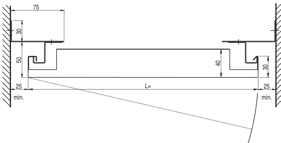
Käytävän katto – yhdellä kasetilla
