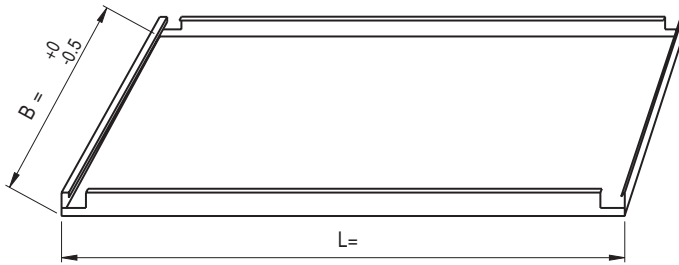
Hook-on Corridor -kasettien mitoituskuvat
