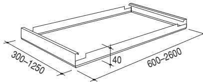
Hook-on-Corridor kasettien mitoitus
