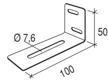
Seinäkannake CC-13. (vaihtoehtoisesti L-lista 75 x 30 mm)
