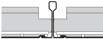
Leikkaus kannatinlistan kohdalta
