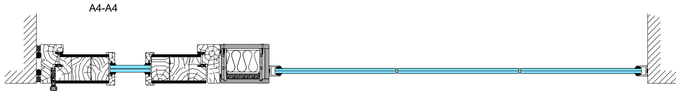
Lasiaukollinen ovi ulosaukeva, sähköpieli
