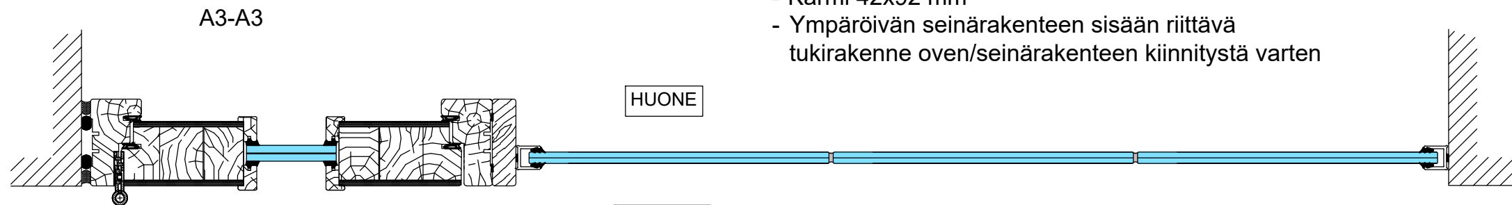
Lasiaukollinen ovi ulosaukeva, apukarmi KÄYTÄVÄ
