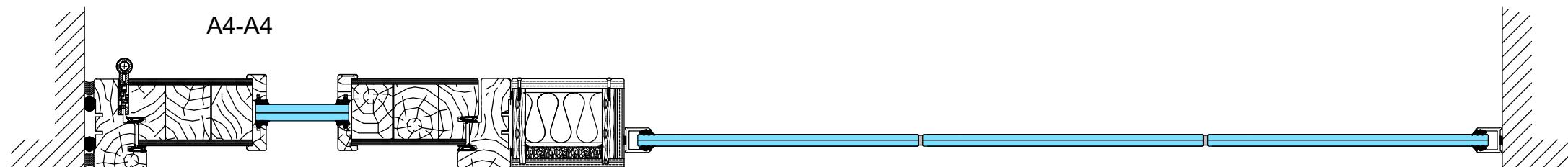
Lasiaukollinen ovi sisäänaukeva, sähköpieli
