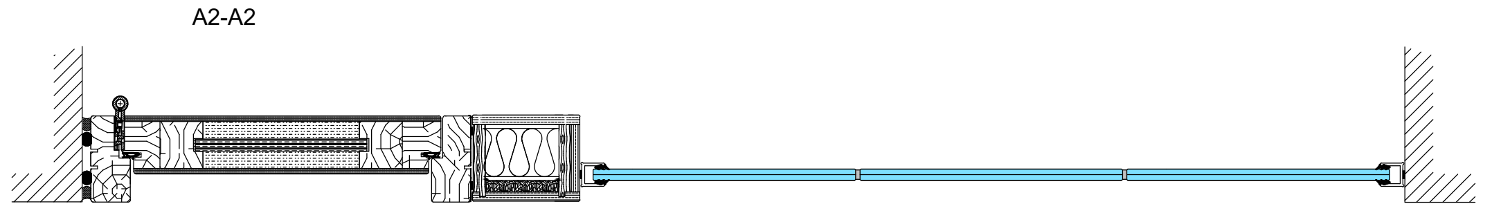
Umpiovi sisäänaukeva, sähköpieli
