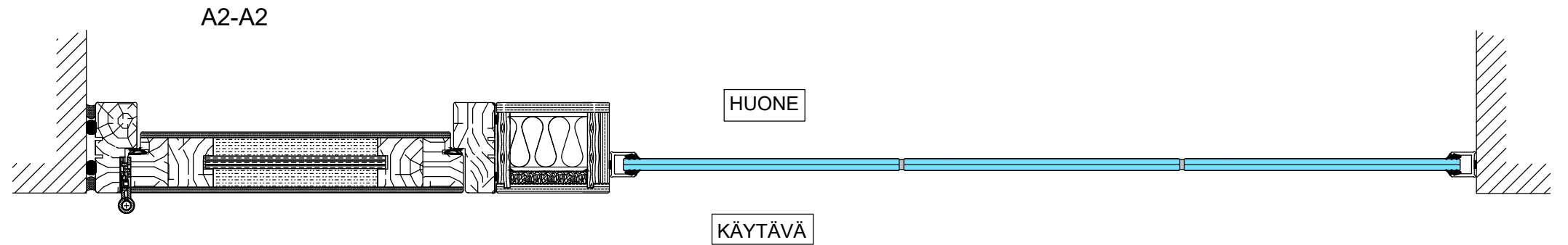
Umpiovi ulosaukeva, sähköpieli
