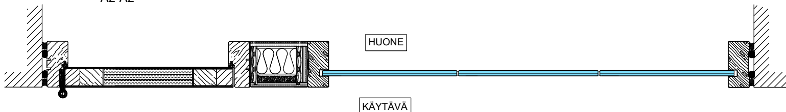
Umpiovi ulosaukeva, sähköpieli
