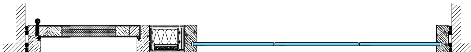
Umpiovi sisäänaukeva, sähköpieli
