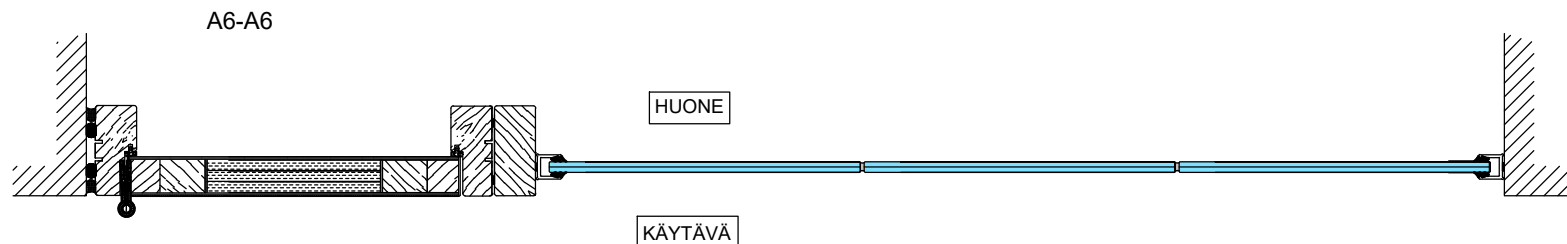
Umpiovi ulosaukeva, apukarmi
