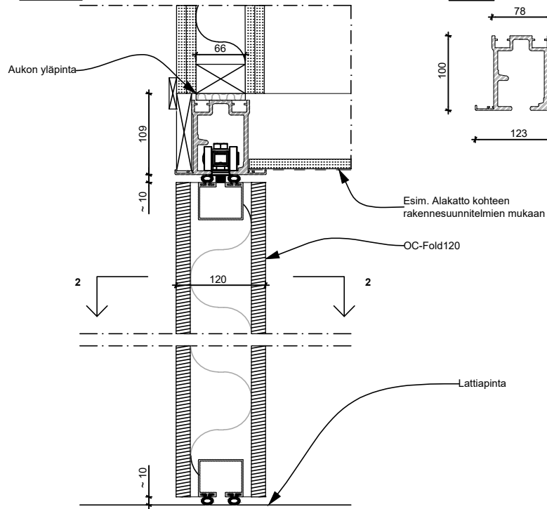
Leikkaus 1-1
